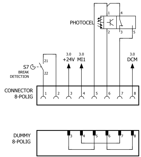
PLC - PHOTOCEL PLC - CBT42
